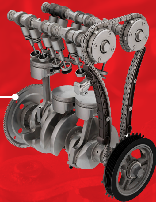
3-циліндровий рядний двигун
