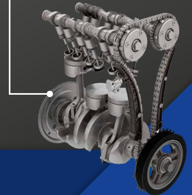
3-циліндровий рядний двигун
