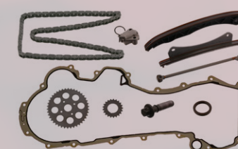
febi 49722 підходить до: Alfa Romeo, Chevrolet, Citroën, FIAT, Ford, Lancia, Opel, Peugeot, Suzuki, Vauxhall (дизельний ДВЗ) Дотримуйтесь інструкцій з монтажу.
