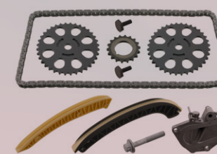
febi 30607 підходить до: Seat, Škoda, VW (бензиновий ДВЗ) Дотримуйтесь інструкцій з монтажу.
